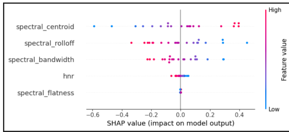
(a) Shap global espectrales
